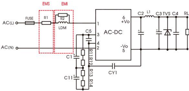
推荐电路 1
