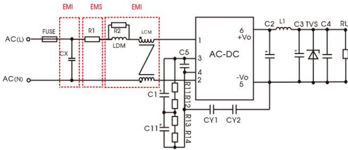
推荐电路 2
